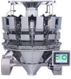
ÇOK KEFELİ TERAZİLER MULTI-HEAD SCALES
